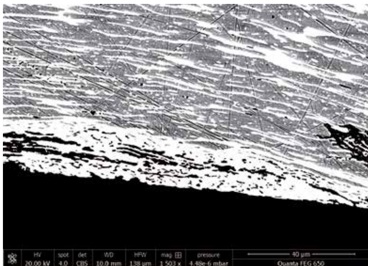
1. SEM/EDX-foto med backscatter-detektor i ett SEM/EDX-mikroskop (FEG650). Mynt från Karl XII, 1 öre 1705, tvärsnitt. De ljusa ytorna är silver och de mörka koppar. Det silvverrika yt-skiktet (med 69% silver) för detta mynt är cirka 20 µm (0.02 mm); jämför med skalan längst ned till höger i bilden.
