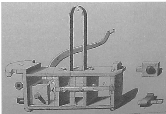
4. Så kallad myntsax. Vid denna maskin arbetade "klipparna" med att stansa ut myntplattor ur koppartenarna.
