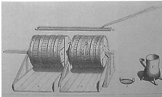
5. "Glögg- och skurarna" skötte bland annat skurtunnorna. \frac{1}{2} skeppund myntplattor fick rotera tillsammans i varje skurtunna för att nöta bort klippgrader etc.
