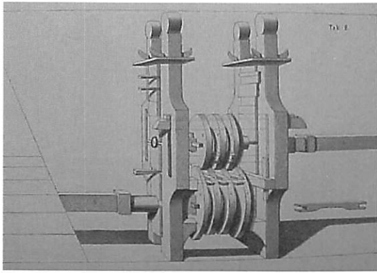
3a och b. Skär- och valsverk i Avesta enligt Anton von Swab 1723.
