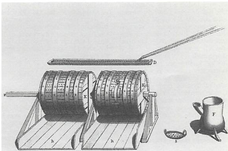
2. S.k. skurtunna använd i Avesta. Denna teckning utförd av Anton Swab år 1723 finns publicerad under rubriken "En kort berättelse om Afwesta Crono-bruk" i NM IX.
