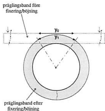
Bild 3. Myntbildens förlängning vid fixering/böjning runt råvalsen.
