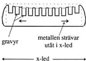
Bild 6. Präglingens bandets utseende efter fixering/böjning runt rävlsen (genomskärning).
