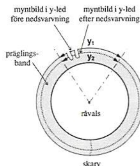
Bild 2. Myntbildens minskning i y -led vid präglingsbandets nedsvarvning.
