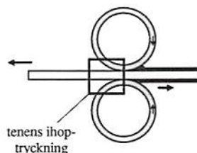
Bild 5. Tenens ihoptryckning vid präglning.
