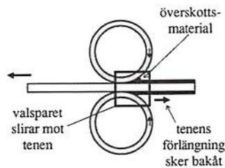
Bild 4. Valsparets slirning.
