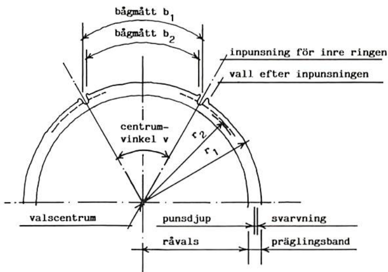
Bild 6. Sektion av en präglingssals före svarvning. (Teckning, J-O Björk)
