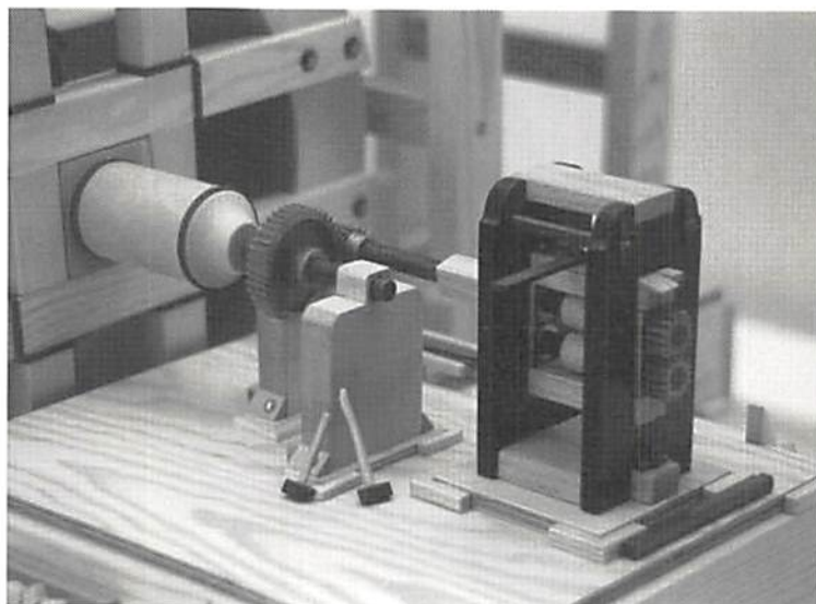
Bild 1. Rekonstruktion av vattendrivet valsverk avsett för myntprägling. Jämför artikeln i SNT 1990 s 4-7. Artikeln och modellerna av S Serrestam. (Foto A Heinonen, Växjö)
