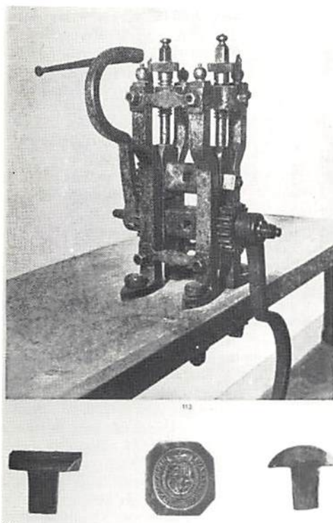
Fig 4. Handdrivet fickvalsverk från 1500-talets senare del. Bilden ur boken "The art craft of coin marking." Förlag Spink & Son 1988.
