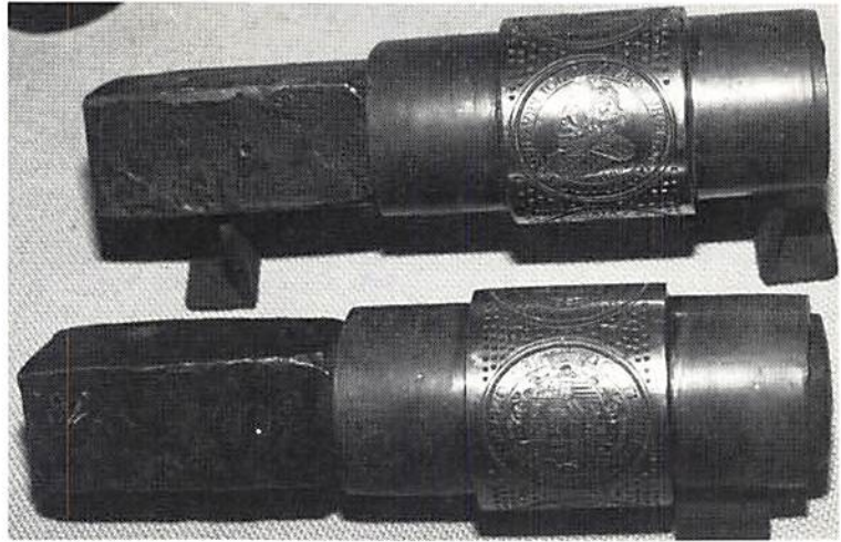
Fig 1. Valspar med två olika talermynt från Hall i Tyrolen 1566. Ur konsthistoriska museets samlingar i Wien. Foto liksom följande Hans Menzinsky.
