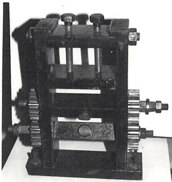
Fig 5. Modell i naturlig storlek (ca 1 m hög) av handdrivet fickvalsverk. Ur konsthistoriska museets samlingar, Wien.
