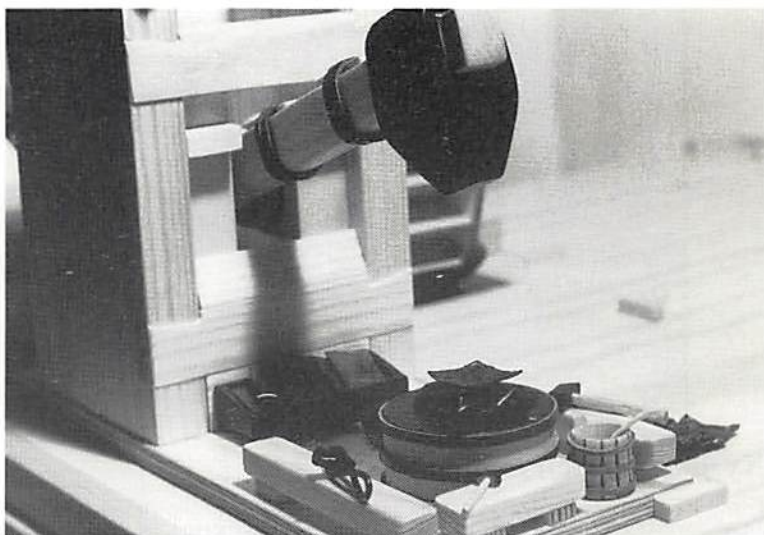
6. Detaljbild av stämpelhammaren sedd snett framifrån. Nedanför hammaren de fyra karlarnas arbetsplats med alla de verktyg som de hade till sin hjälp vid arbetet.
