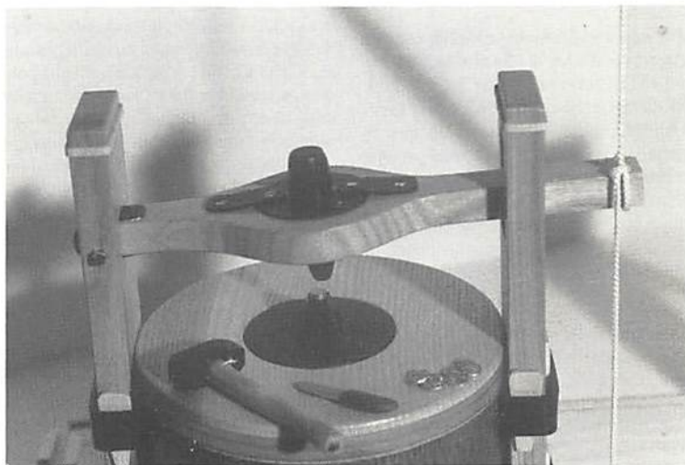
4. Detaljbild av slaggverkets uppbyggnad. Två stolpar fastsatta med kilar i en cylinder. Den övre stampen fastsatt i överarmen (fiolen) som är kopplad med en lina till hävarmen och pedalen. I centrum av cylindern ett städ med en pyramidformad understamp.
