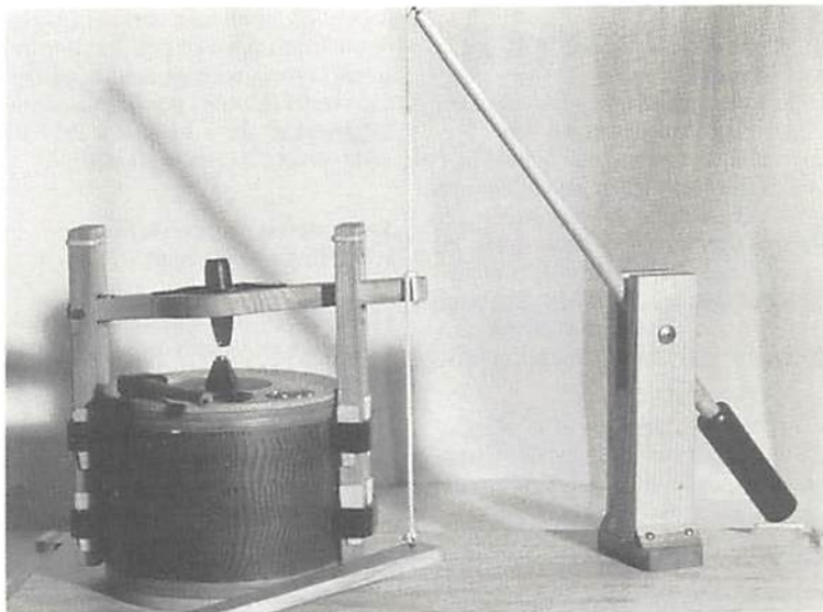
3. Manuellt slaggverk använt vid myntverket i Avesta. En man i sittande ställning passade in myntämnet på understampen, trampade på pedalen så överstampen gick ned mot den undre. En man stående på andra sidan slog ett kraftigt slag med handslaggen mot överstampen, varefter man hade ett präglat mynt.
