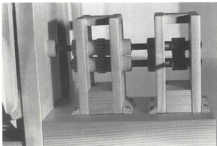
2. Detaljbild av valsverkets uppbyggnad med präglingsvalsar och kugghjul förbundna med de axlar som drev valsarna runt. Stora kopparmynt, typ Kristinas och Karl XI:s 1-öringar, förutsäts på modellen ha fem myntbilder graverade på valsens. Det skulle ge valsens en diameter på cirka 8 cm.
