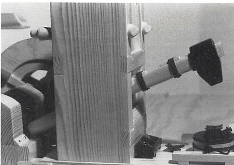
5. Vattendrivet slägghverk av den typ som användes på 1700-talet i Avesta för stämpling av plåtmynt. Bilden visar stämplinghammaren från sidan med hjulet som lyfter hammaren. Det hela är via hjulstocken förbundet med vattenhjulet. Ett tryck på över 600 kilo krävdes för att lyfta hammaren.
