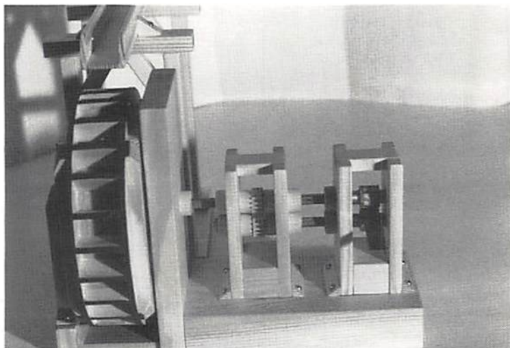
1. Rekonstruktion av vattendrivet valsverk. Valsverket var en effektiv präglingsmetod som genom åren kom att producera stora mängder kopparmynt i Sverige. Det var i det långa loppet alltför dyrbart med ständiga byten av valsarna som fort blev uppslitna eller på annat sätt skadade. Foto: (liksom följande) L. Svensson Vexjö.
