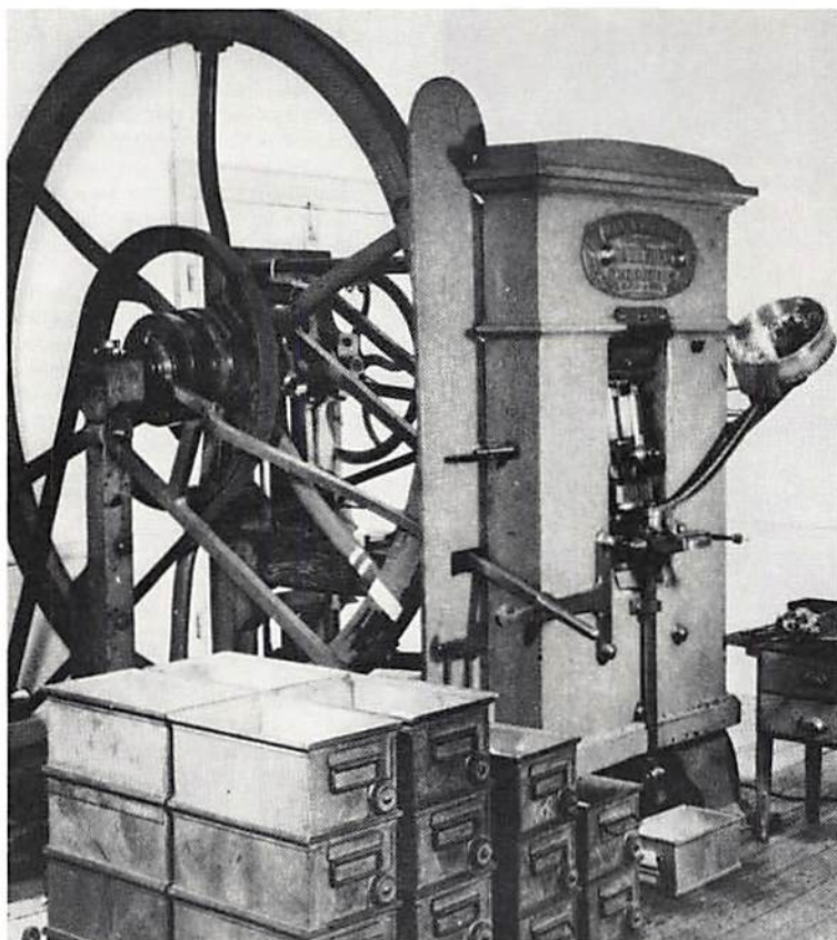
Fig 5. Präglingmaskin från 1857, med tiden den äldsta i bruk (till 1972) och kallad "mormor". Numera uppställd i Eskilstuna museer. Foto ATA 1950.
