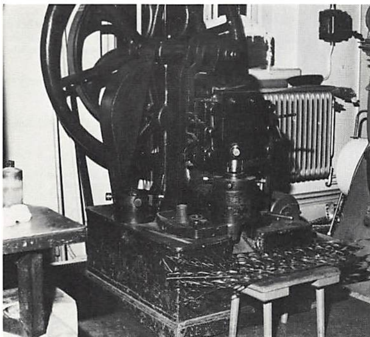
Fig 7. Kombinerad sax och uthuggningspress för medaljplattor. Maskinen troligen från 1860-70-talen. Foto G. Hildebrand, ATA (1972).
