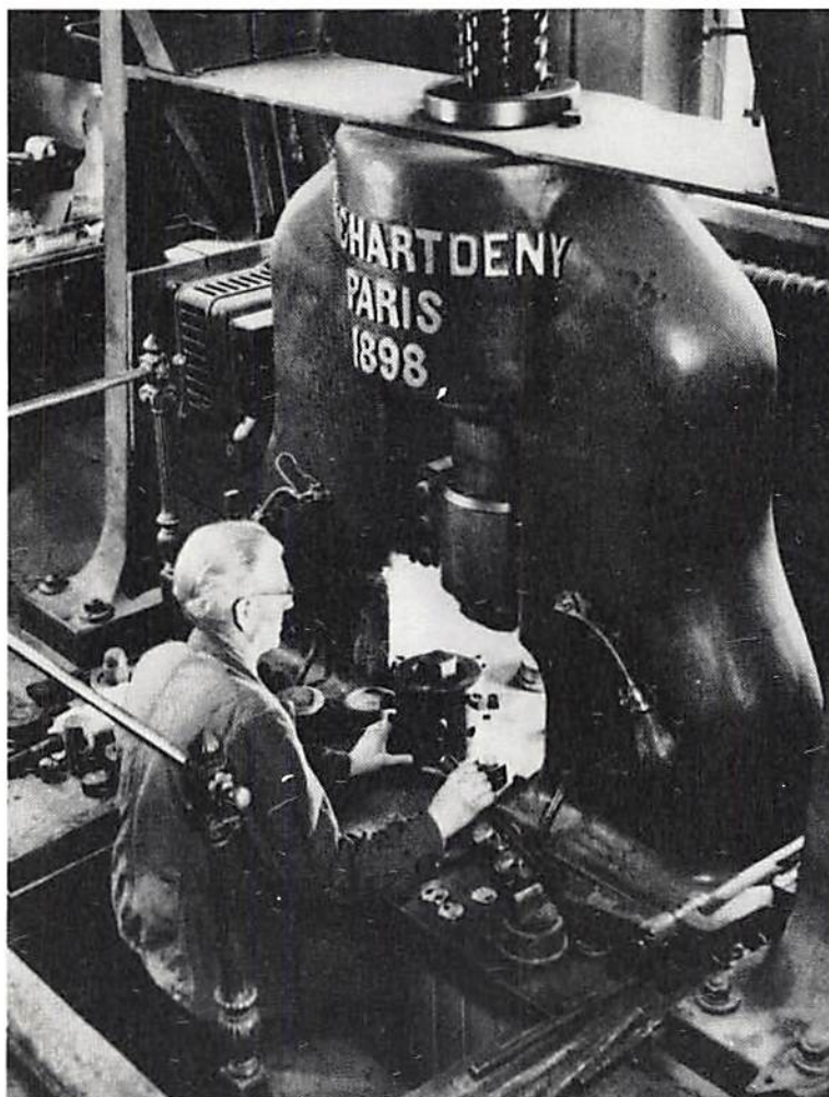
Fig 8. Fransk medaljpräglingsmaskin från 1898, i bruk på myntverket fram till flytningen 1974. Den som användes vid reportaget 1889 var alltså något "omodernare". Foto G. Hildebrand, ATA (1972).
