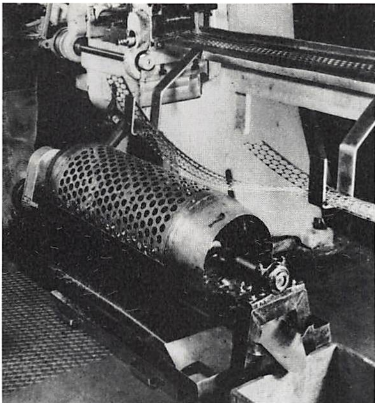
Fig 3. Så här såg det ut när myntplattor stansades ut med hjälp av en "punchmaskin" (1950), ett arbete som drevs maskinellt också under reportaget 1889. Myntverket upphörde att tillverka egna myntdämn av brons och nickel 1962, silver 1968. Foto ATA 1950.
