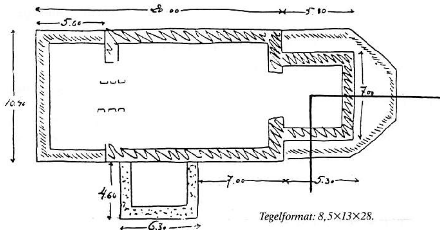
Fig 1. Plan av Gestad gamla kyrka efter utgrävningen 1917. Den sydöstra delen av koret är markerad.
