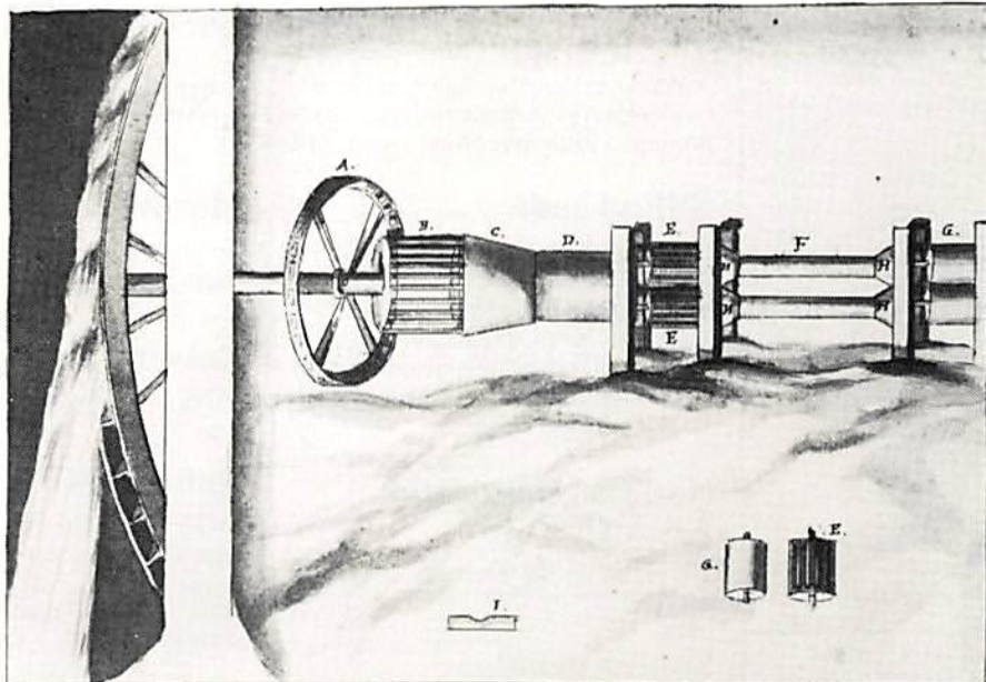
A. Rugghjul. B. Trilla. C. Flygh. D. Valsbom. E. Valsghjul med skafflor. F. Valsbom. G. Sje våt Valsghjul. H. Flygh. I. Fanna. ~ ~ ~
