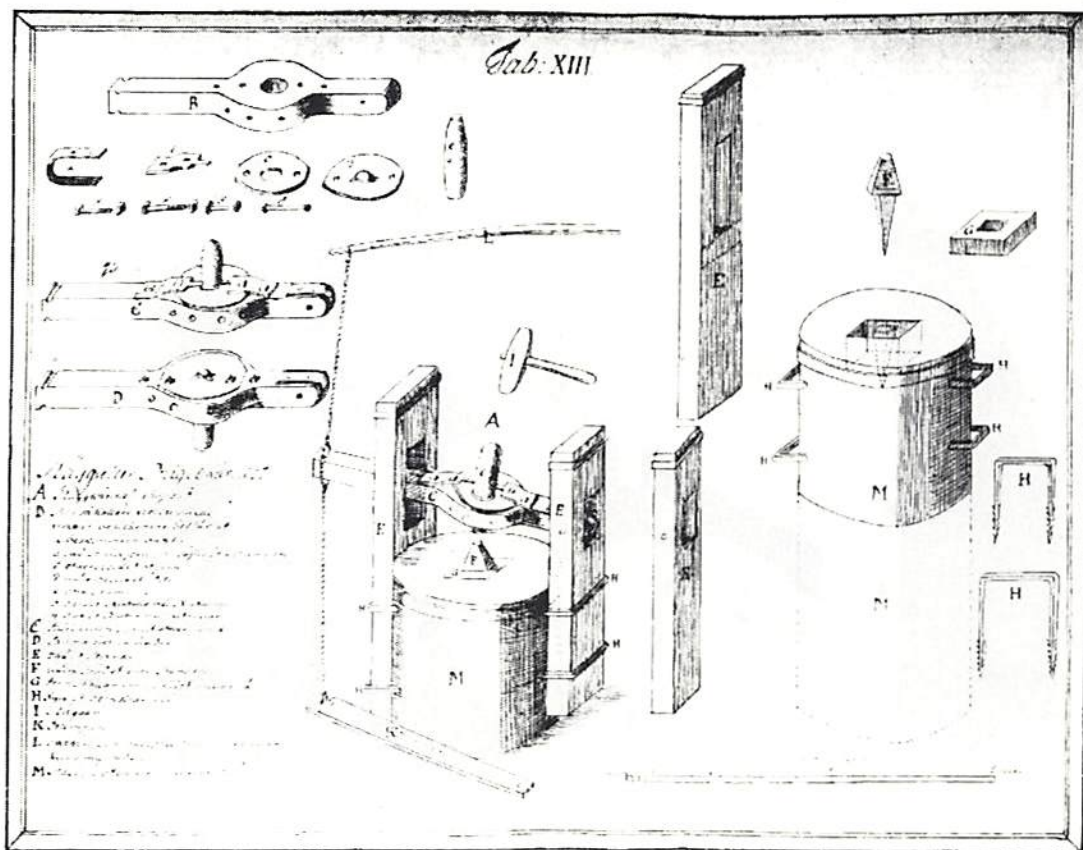
10. Ett s k släggverk, använt under 1700- och början av 1800-talen (1715–1832 vid Avesta myntverk. Detta var en förbättring av metoden att prägla för hand. När man 1715 upphörde att använda valsverk vid Avesta var detta tekniskt sett en tillbakagång, men valsverkspräglingen var komplicerad och arbetskraften billig.
