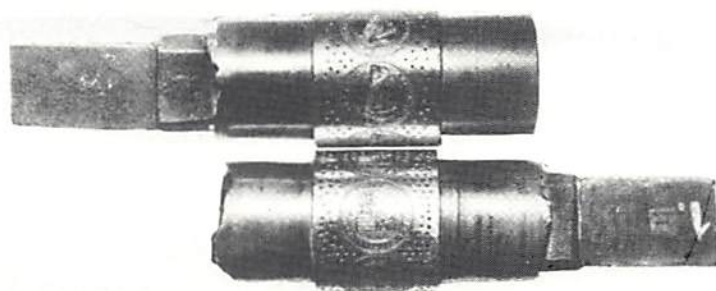
4. Verktyg för valsverksprägling. Bilden visar själva valsarna i en dylik maskin för myntframställning, graverade med flera på varandra följande stampar till österrikska talrar från 1566. Mellan valsarna infördes sedan metallen i ett långt band; sedan den fått bild på bägge sidor, utklipptes mynten (nedan). Från myntverket i Hall, Tyrolen; numera förvarade i Wien.
