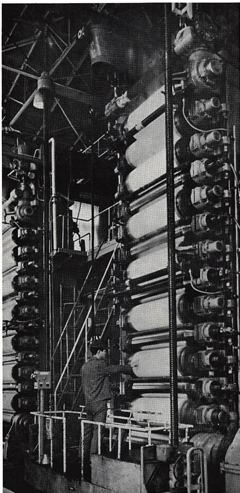
Ark med tryckta sedlar glättas i dessa pressar.
