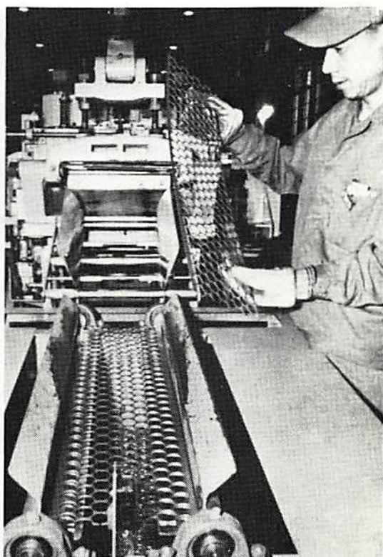
Myntämnen görs i en speciell ämnesskärarmaskin.
