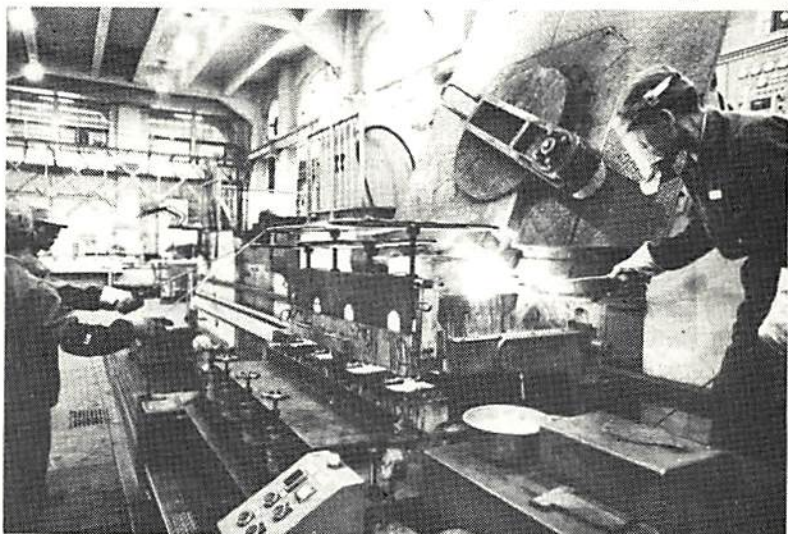
Att göra plantsen är det första steget i mynttillverkning. (Forts. nästa sida)
