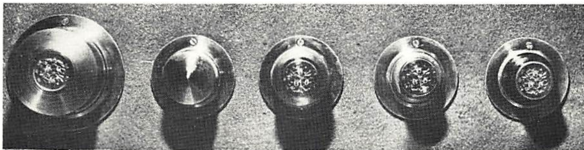
Myntstämpeln som är fäst vid stampen är gjord via en komplicerad process. Från vänster till höger återfinns: huvudstämpeln, stålstämpeln, stålstämpeln efter press, efter utformning och den slutgiltiga stämpeln.
