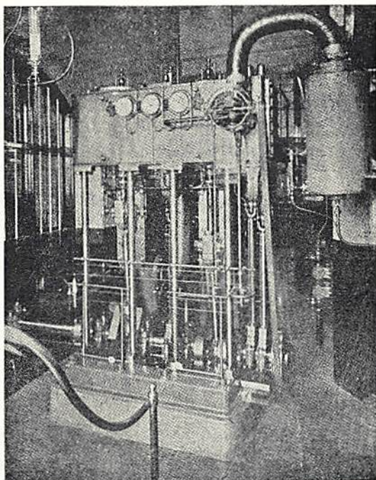
Ångmaskinen
