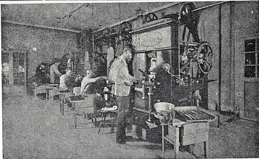
Maskin för uppstukning af kanten å myntplattorna (ovan)
