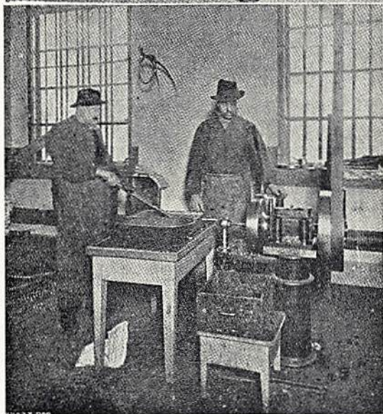
Maskin för uppstukning af kanten å myntplattorna (ovan)
